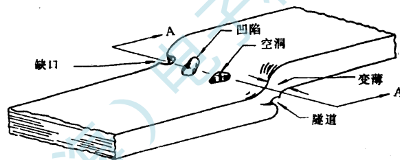
金属化在氧化层台阶处的各种典型缺陷
