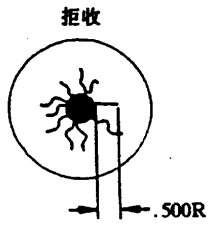
图 2071-1 超过引出端至外壳距离一半的径向裂纹
