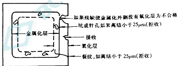
图 2073-3 有划片槽的氧化层钝化器件
