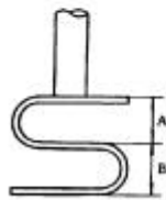
如果 A 或 B 小于设计压缩高度的 50% 不合格 图 2074-9“S”形触须压缩高度
