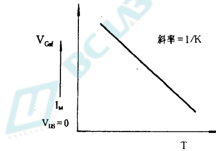
图 3104-5 V_{GSF} 与 T_J 关系的曲线实例
