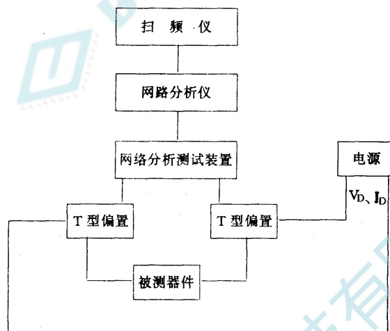
图 3570—1 S 参数测试系统
