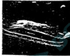
图 2077-18 (5000X)接触窗口区一般金属化的剥离或翘起(不合格)
